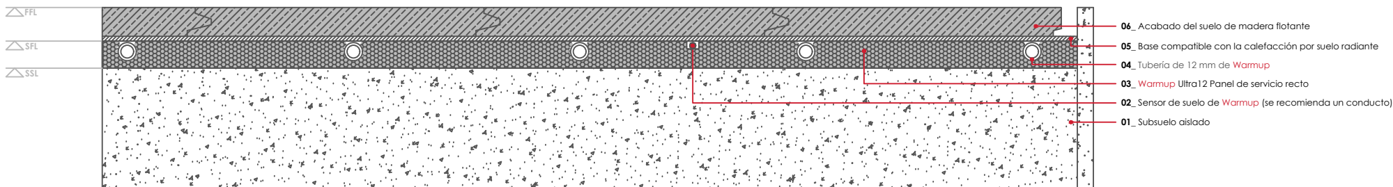
WARMUP SISTEMA ULTRA12. Acabado del suelo de madera flotante
