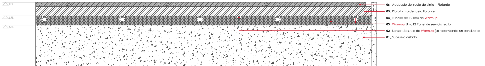
WARMUP SISTEMA ULTRA12. Acabado del suelo de vinilo - Flotante
