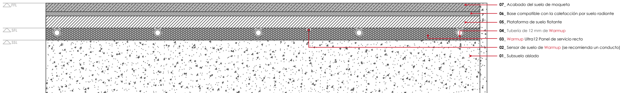
WARMUP SISTEMA ULTRA12. Acabado del suelo de moqueta
