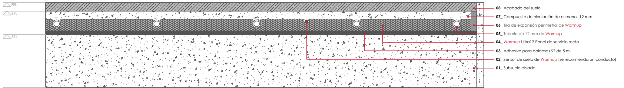
WARMUP SISTEMA ULTRA12. Detalle estándar
