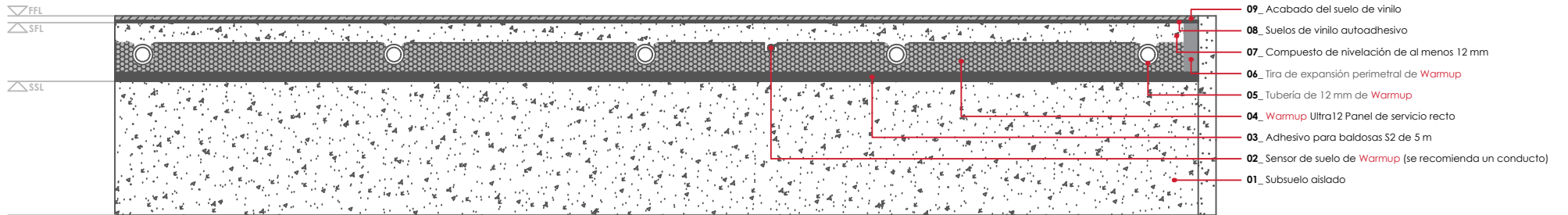
WARMUP SISTEMA ULTRA12. Acabado del suelo de vinilo - Pegado
