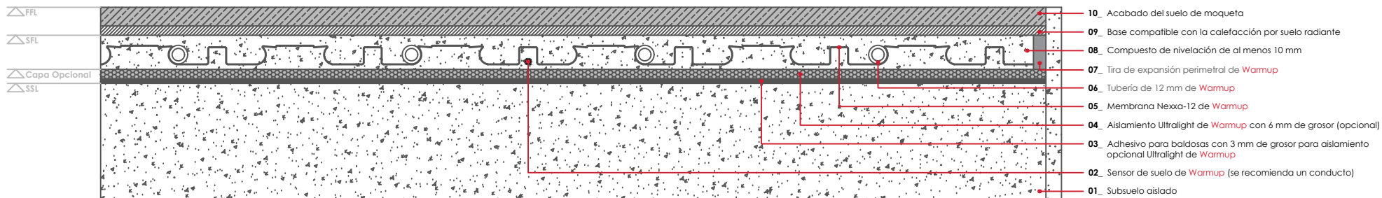
WARMUP SISTEMA NEXXA12. Acabado del suelo de moqueta
