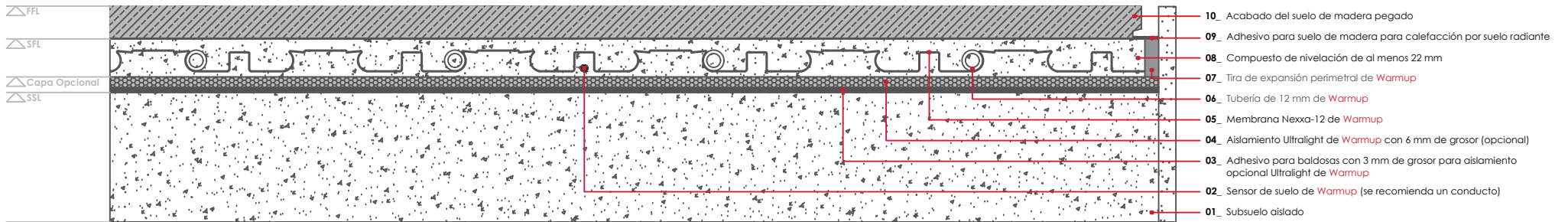
WARMUP SISTEMA NEXXA12. Acabado del suelo de madera pegado
