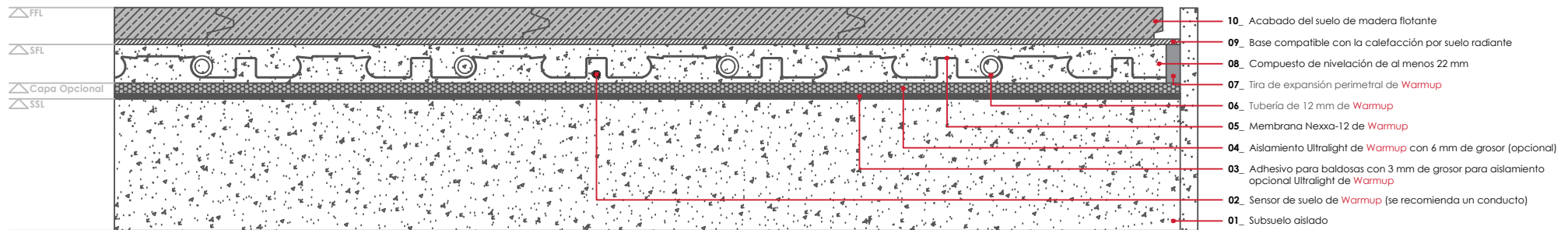
WARMUP SISTEMA NEXXA12. Acabado del suelo de madera flotante
