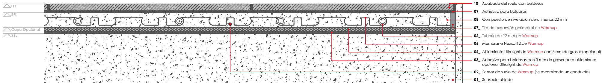
WARMUP SISTEMA NEXXA12. Acabado del suelo con baldosas
