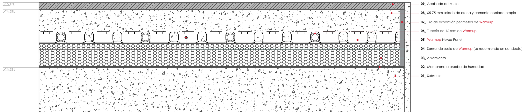
WARMUP SISTEMA NEXXA. Detalle estándar
