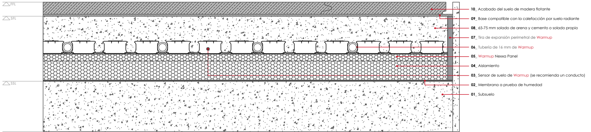
WARMUP SISTEMA NEXXA. Acabado del suelo de madera flotante
