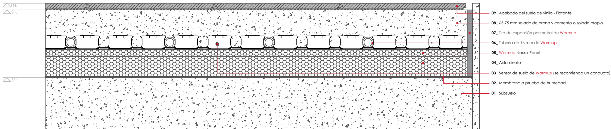
WARMUP SISTEMA NEXXA. Acabado del suelo de vinilo - Flotante
