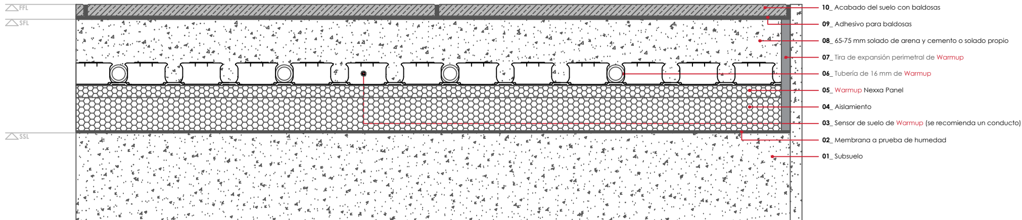
WARMUP SISTEMA NEXXA. Acabado del suelo con baldosas
