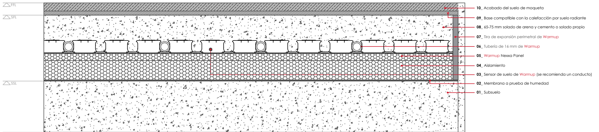
WARMUP SISTEMA NEXXA. Acabado del suelo de moqueta
