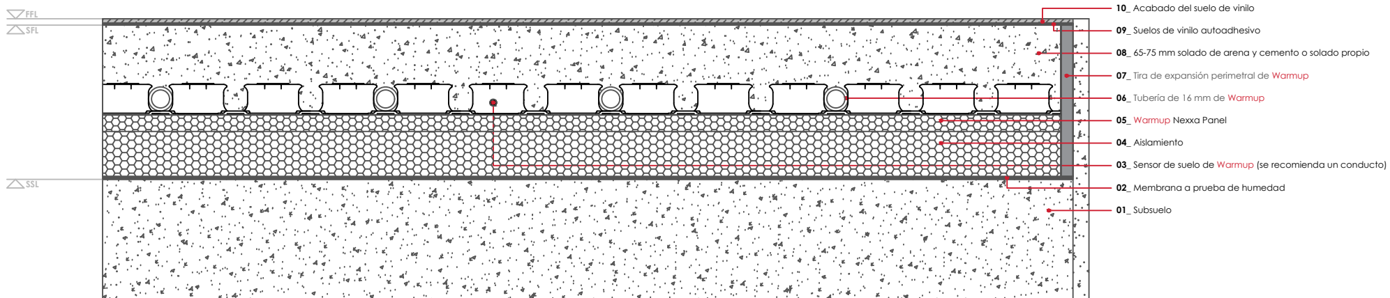
WARMUP SISTEMA NEXXA. Acabado del suelo de vinilo - Pegado
