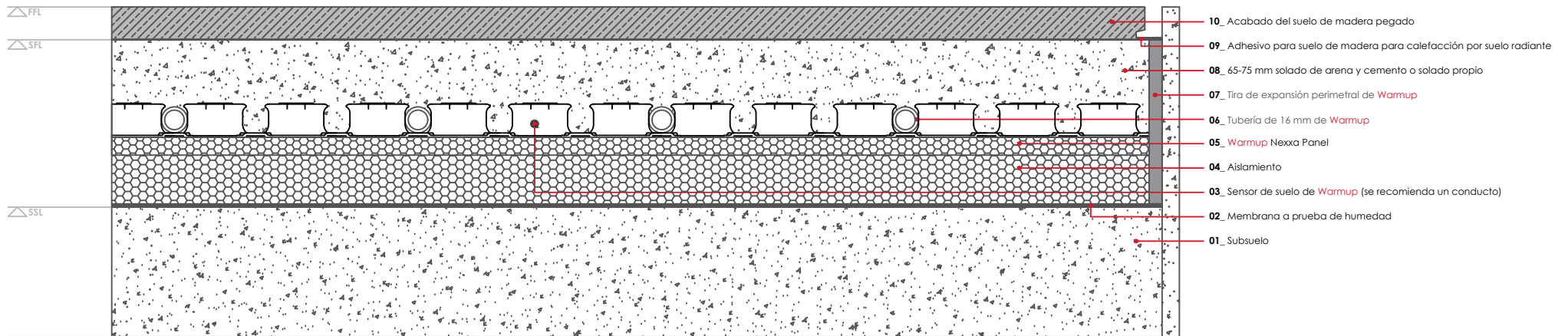
WARMUP SISTEMA NEXXA. Acabado del suelo de madera pegado
